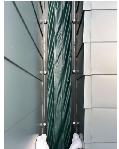
スライドファスナーによる連結
